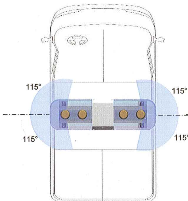
Rampe ORION BF2 (2 feux spéciaux)
