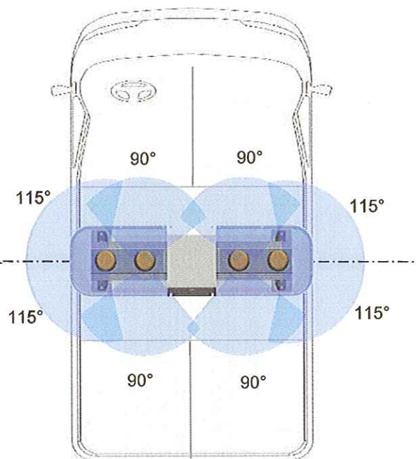
Rampe ORION BF4 (4 feux spéciaux)
